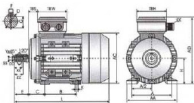
IMB3
