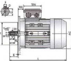
IMB5
