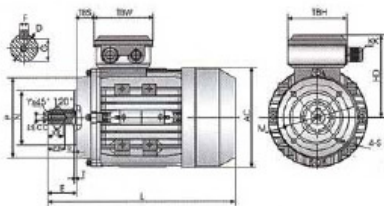
IMB14
